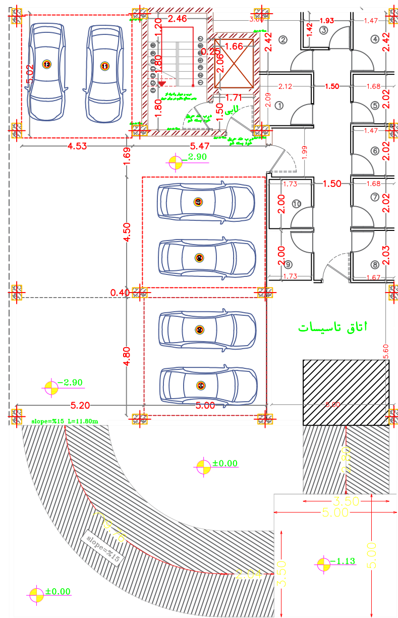
پلان طبقه زیرزمین ۱-
