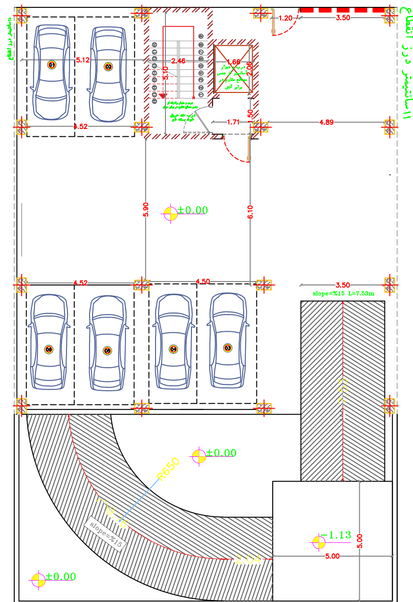
پلان طبقه همگف
